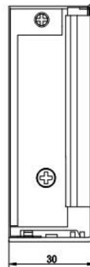
右视图
