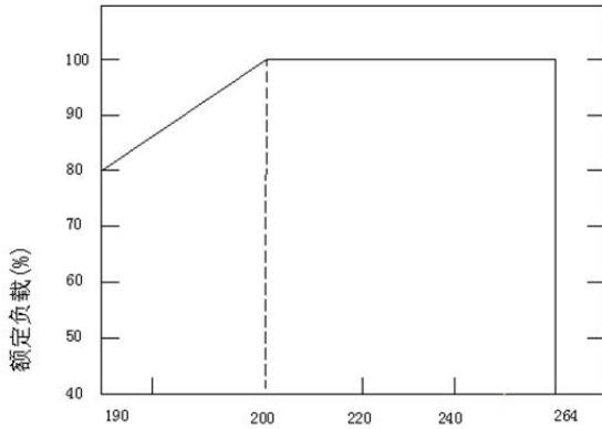
■ 输入电压VS额定功率降额曲线
